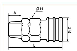
Con filetto maschio tipo SM
