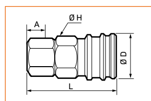
Con filetto femmina tipo SF
